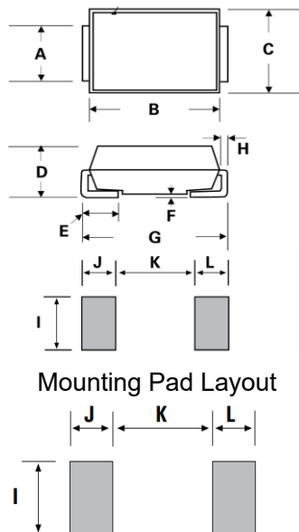
DO-214AA (SMB J-Bend)
